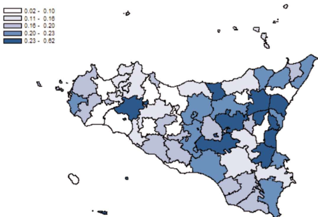
Distribuzione spaziale dei TSD per distretto di residenza (aa 2009-2011)
